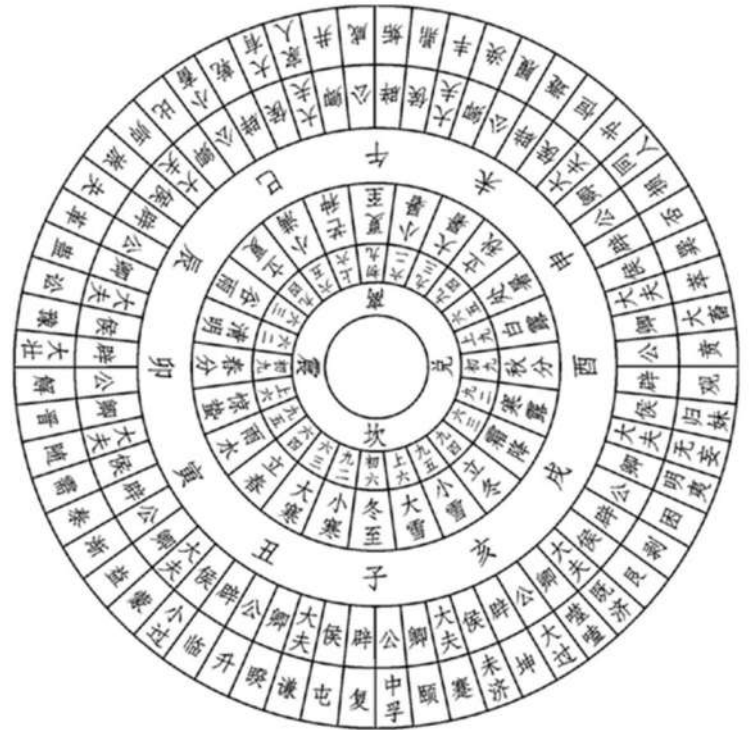
六日七分圖
