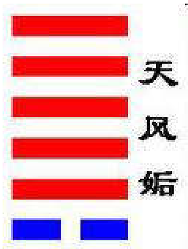
四十四卦
